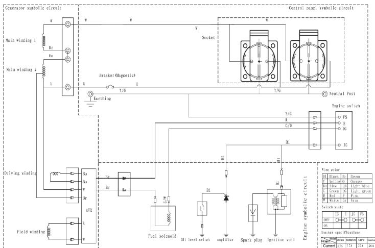
DG401 - Diagrama circuito eléctrico
