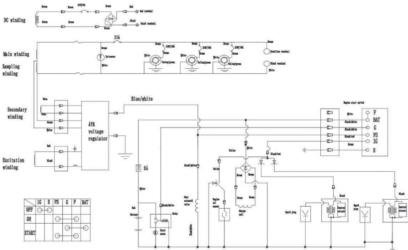
DG121 - Diagrama circuito eléctrico
